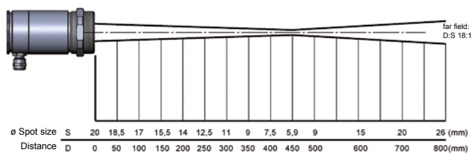
CF4 optics 75:1
