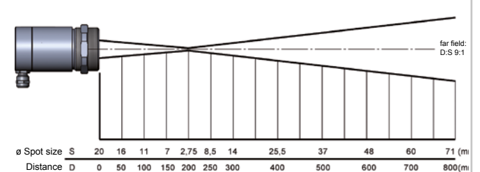
CF3 optics 75:1
